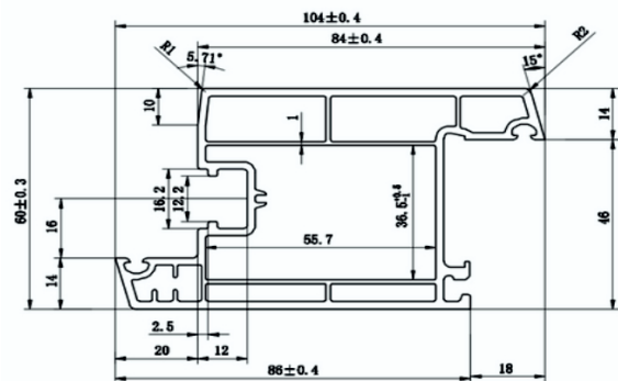
CASEMENT DOOR SASH INWARD
