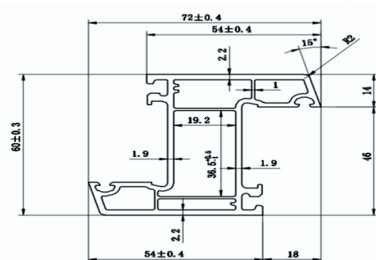
CASEMENT DOOR SASH INWARD
