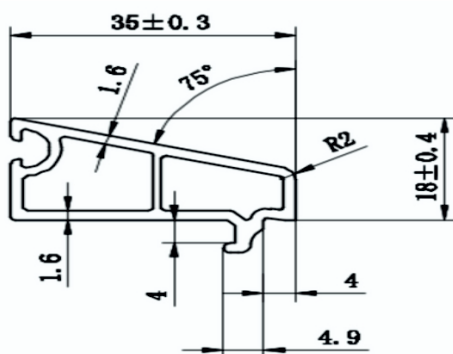
CASEMENT T-MULLION
